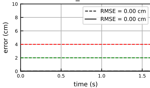
_SAE
