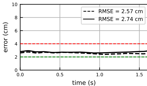
_FME
