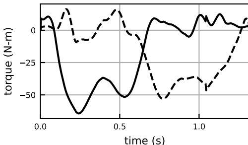
ankle_angle_moment
