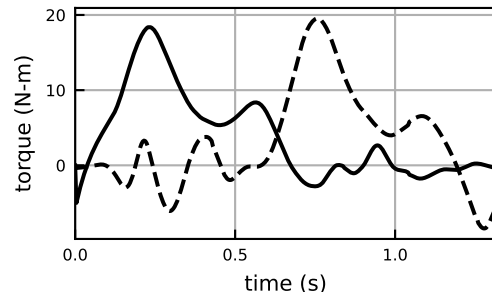
subtalar_angle_moment
