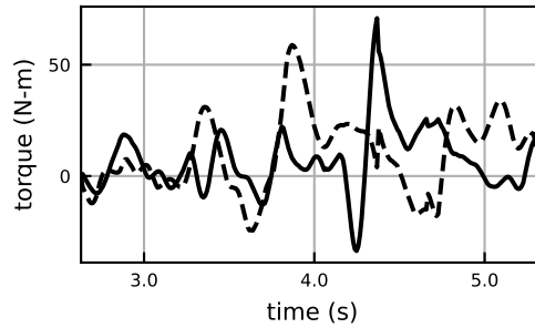
ankle_angle_moment
