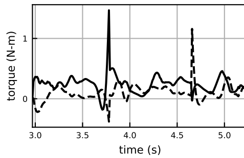
wrist_dev_moment
