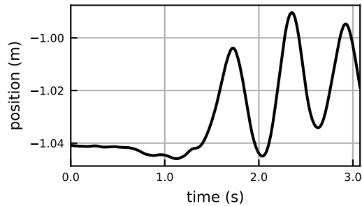
hip_adduction
