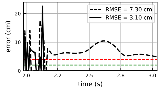
MT5
