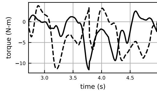
subtalar_angle_moment
