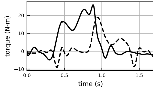
subtalar_angle_moment
