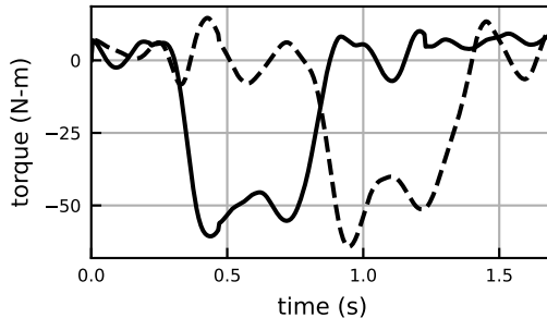
ankle_angle_moment
