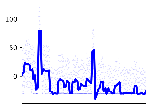
/jointset/hip_l/hip_flexion_l/value
