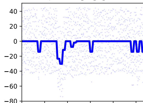
/jointset/radioulnar_r/pro_sup_r/value
