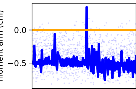
/forceset/grac_r_moment_arm_hip_rotation_r
