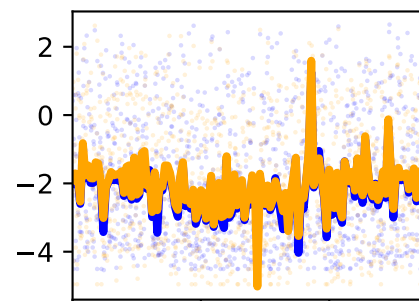
/forceset/glmin3_r_moment_arm_hip_flexion_r
