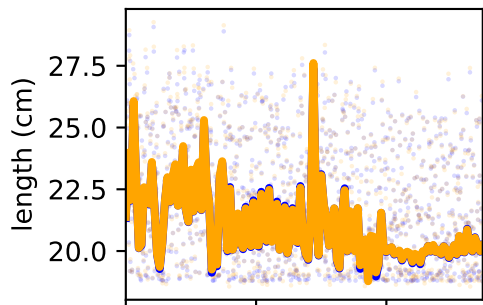
/forceset/glmin1_l_length
