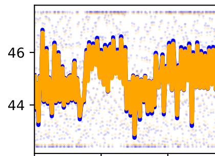
/forceset/gasmed_l_length
