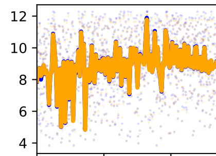
/forceset/glmin3_l_length
