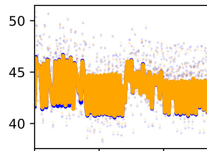
/forceset/bflh_l_length
