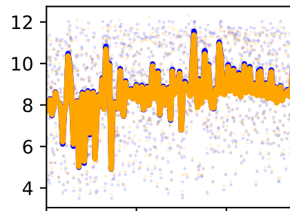
/forceset/glmin2_l_length
