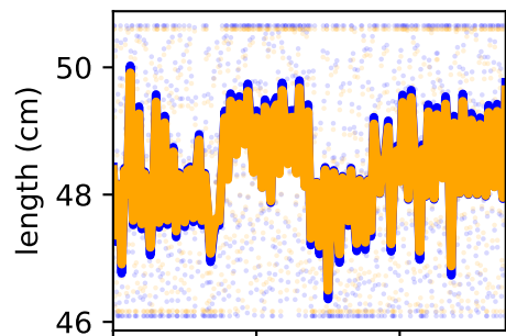
/forceset/gaslat_l_length
