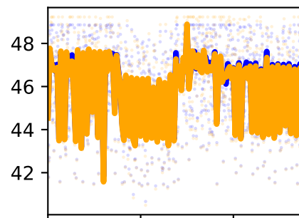
/forceset/glmed1_l_length
