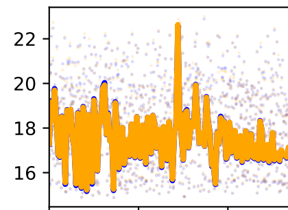
/forceset/glmed2_l_length
