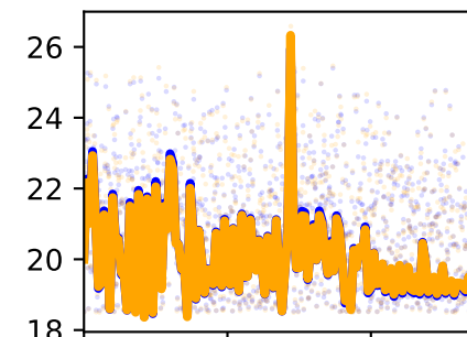
/forceset/glmed3_l_length
