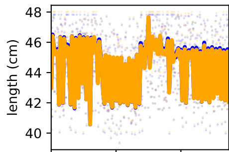
/forceset/glmax3_l_length
