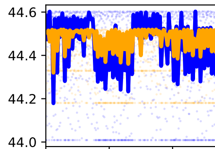
/forceset/glmax2_l_length
