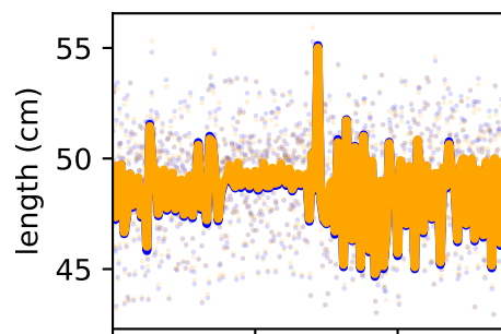
/forceset/semiten_r_length
