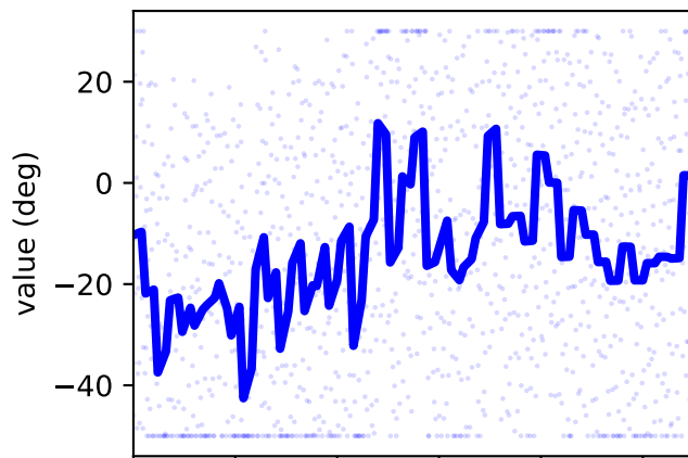
/jointset/hip_l/hip_adduction_l/value
