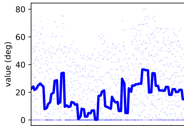
/jointset/hip_l/hip_adduction_l/value
