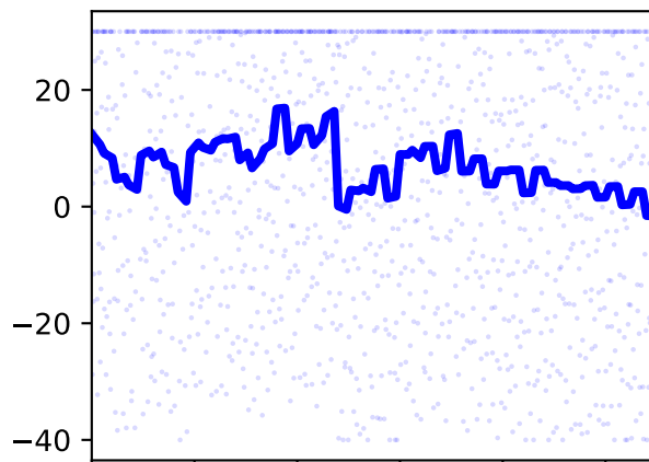
/jointset/hip_l/hip_rotation_l/value
