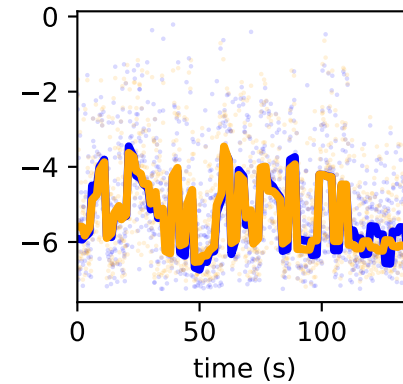
/forceset/glmax1_r_moment_arm_hip_flexion_r
