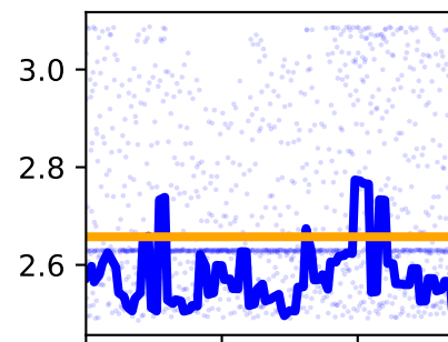
/forceset/glmax1_r_moment_arm_hip_flexion_r
