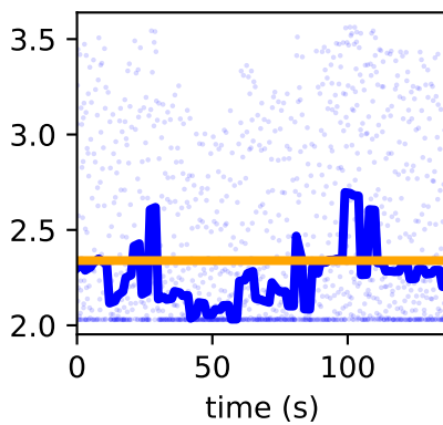
/forceset/gasmed_r_moment_arm_knee_angle_r
