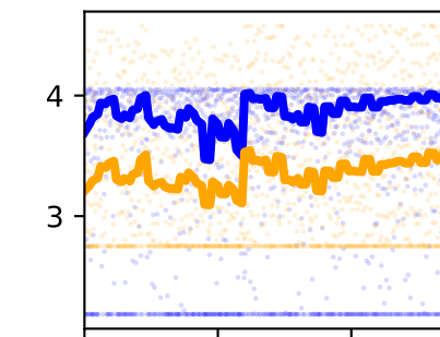
/forceset/gaslat_r_moment_arm_knee_angle_r
