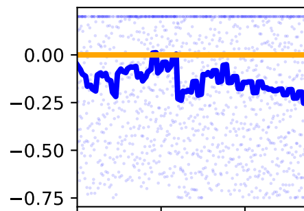
/forceset/gasmed_r_moment_arm_knee_angle_r
