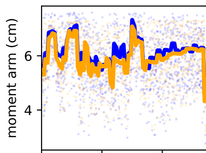
/forceset/bflh_r_moment_arm_hip_rotation_r
