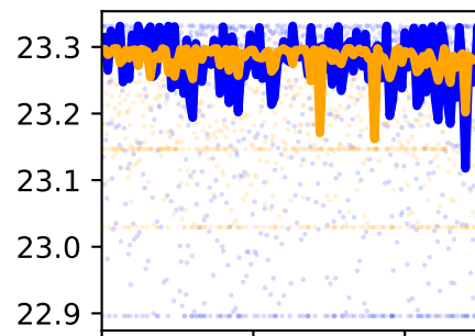
/forceset/recfem_l_length
