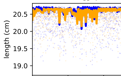
/forceset/iliacus_r_length
