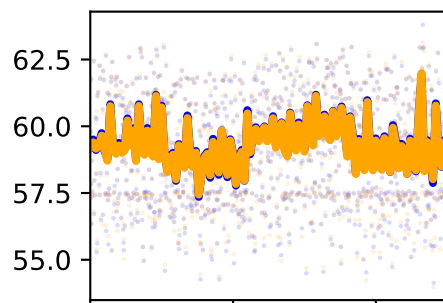
/forceset/recfem_r_length
