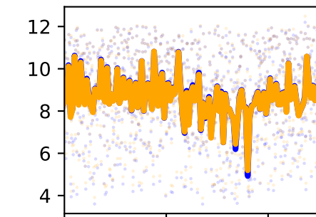
/forceset/glmin2_l_length
