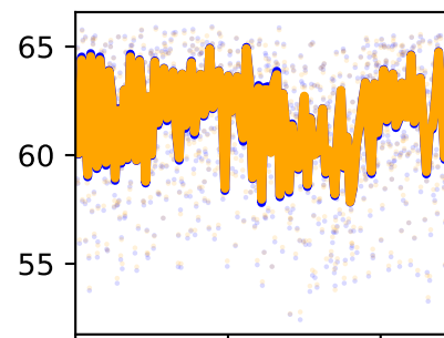
/forceset/tfl_l_length
