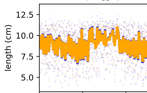
/forceset/glmin1_r_length
