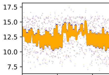
/forceset/glmed1_r_length
