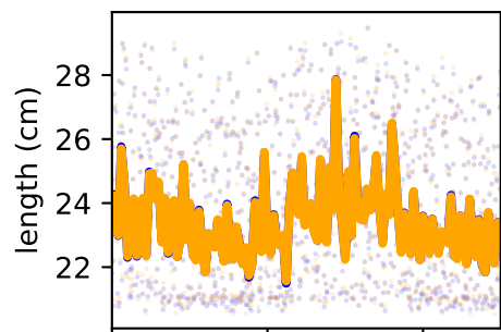
/forceset/glmax3_l_length
