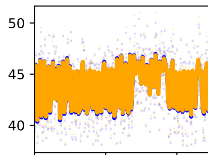
/forceset/bflh_l_length
