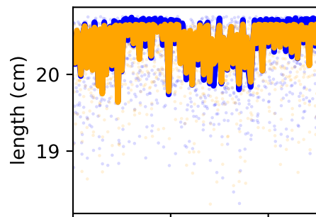
/forceset/psoas_l_length
