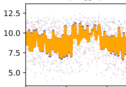
/forceset/glmin2_r_length
