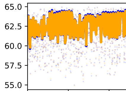
/forceset/tfl_l_length
