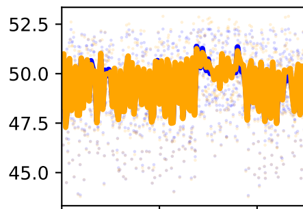
/forceset/glmed1_l_length
