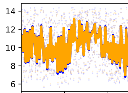
/forceset/glmed3_r_length
