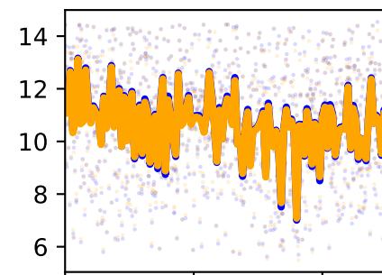
/forceset/glmed3_l_length
