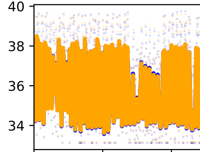
/forceset/vaslat_l_length
