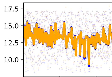
/forceset/glmed2_l_length
