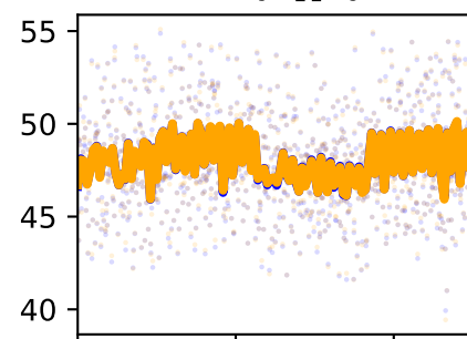
/forceset/grac_r_length
