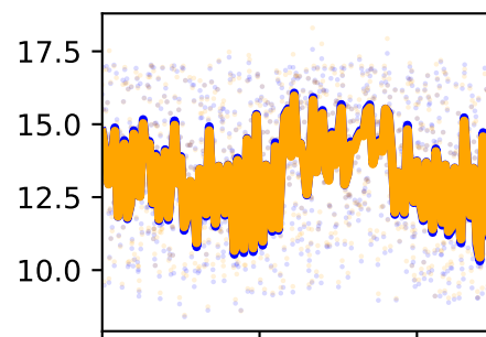
/forceset/glmed2_r_length
