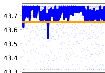
/forceset/perlong_r_length
