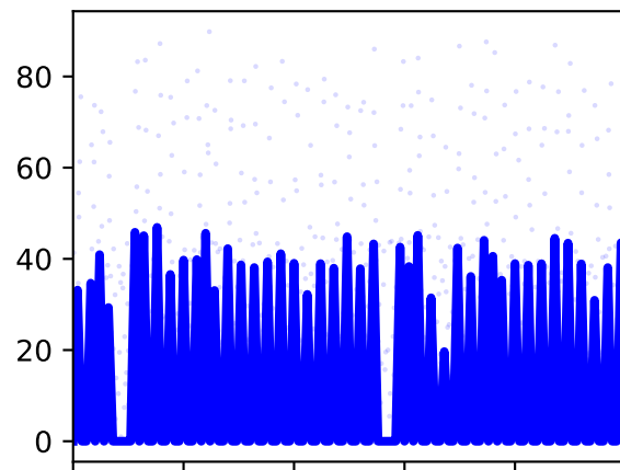
/jointset/radioulnar_l/pro_sup_l/value
