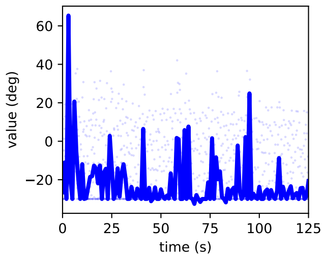
/jointset/hip_r/hip_flexion_r/value
