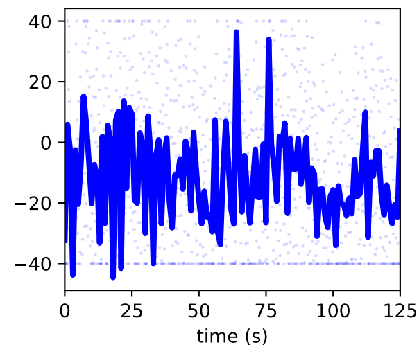
/jointset/hip_r/hip_rotation_r/value
