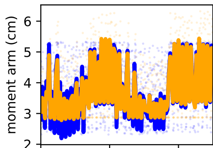
/forceset/grac_l_moment_arm_knee_angle_l
