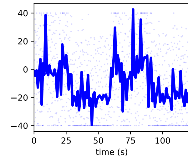
/jointset/hip_r/hip_rotation_r/value
