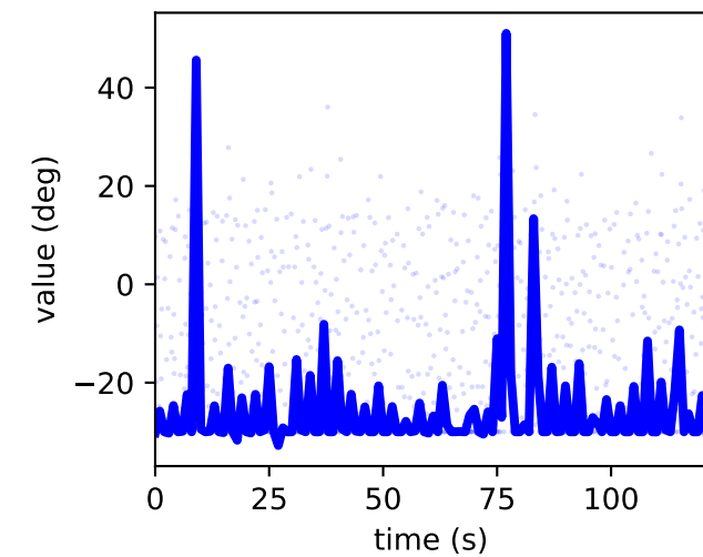
/jointset/hip_r/hip_flexion_r/value
