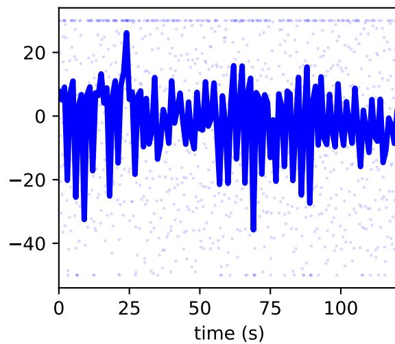
/jointset/hip_r/hip_adduction_r/value
