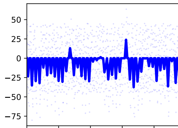
/jointset/radioulnar_r/pro_sup_r/value
