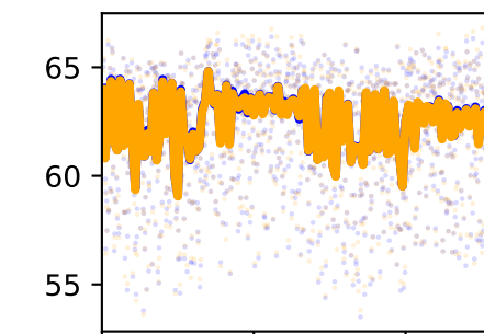
/forceset/tfl_l_length
