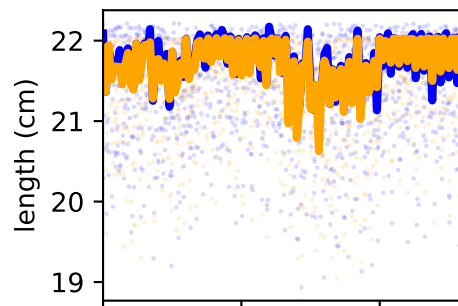
/forceset/psoas_l_length
