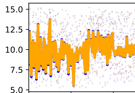
/forceset/grac_r_length
