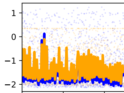
/forceset/glmax3_l_moment_arm_hip_rotation_l
