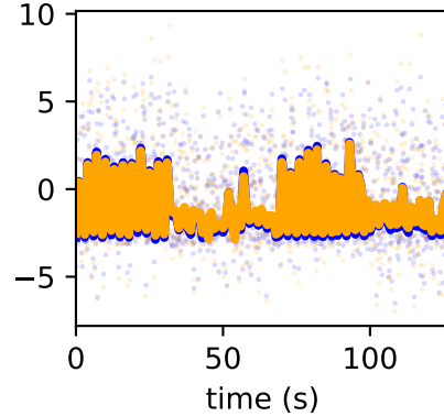
/forceset/glmed1_l_moment_arm_hip_rotation_l
