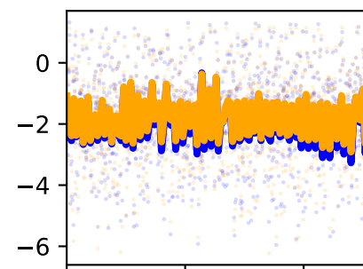
/forceset/glmax1_l_moment_arm_hip_adduction_l
