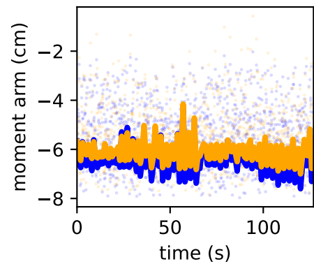
/forceset/glmed1_l_moment_arm_hip_adduction_l
