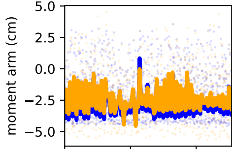
/forceset/glmax1_l_moment_arm_hip_rotation_l
