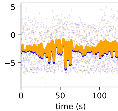
/forceset/glmed2_l_moment_arm_hip_flexion_l
