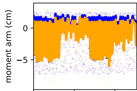
/forceset/glmax3_l_moment_arm_hip_flexion_l
