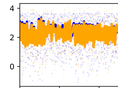
/forceset/bflh_l_moment_arm_hip_adduction_l
