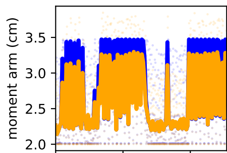
/forceset/gasmed_l_moment_arm_knee_angle_l
