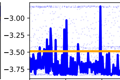
/forceset/gaslat_l_moment_arm_ankle_angle_l
