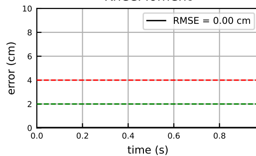
KneeMoment
