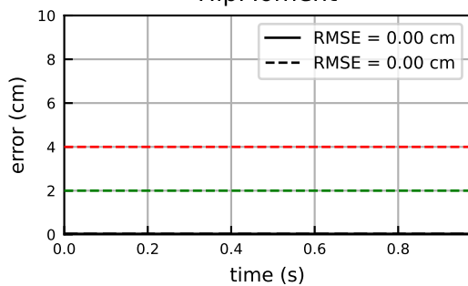
HipMoment
