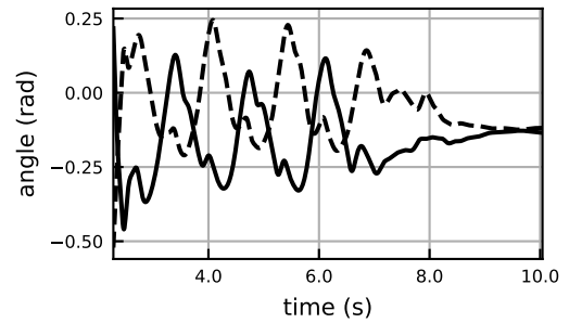
subtalar_angle
