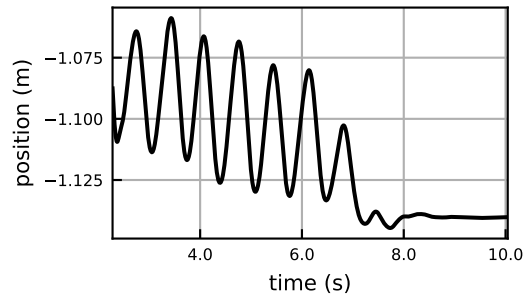
hip_adduction
