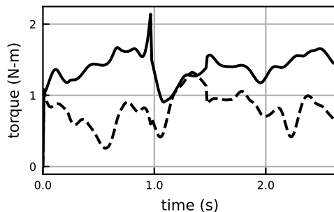
wrist_dev_moment
