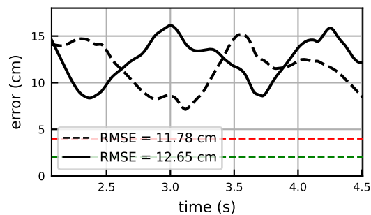
MT5
