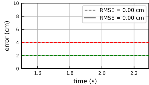
HipForce
