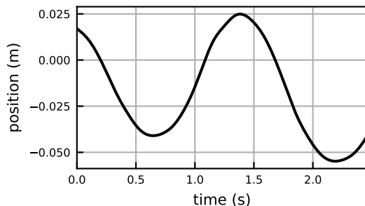
hip_flexion
