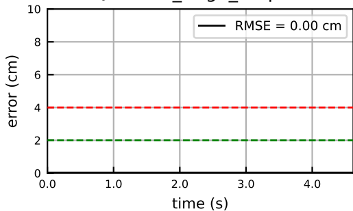
QTMMMod_trunk_t8
