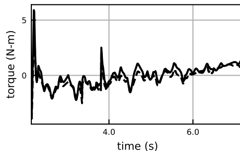
wrist_dev_moment
