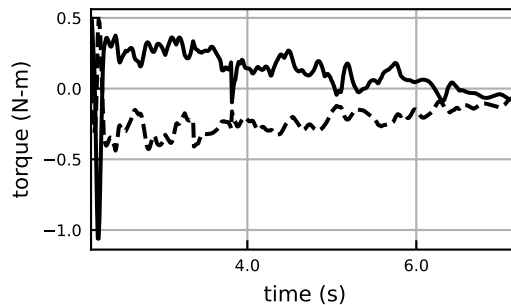
wrist_dev_moment
