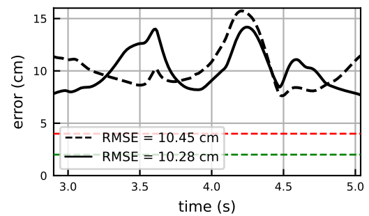
MT5
