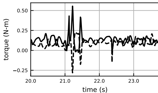
wrist_dev_moment
