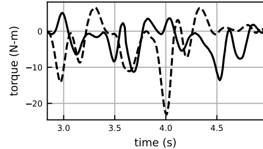
subtalar_angle_moment
