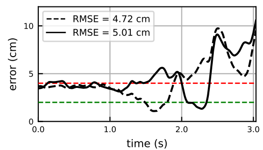
TOE
