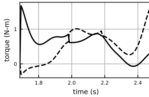
wrist_dev_moment
