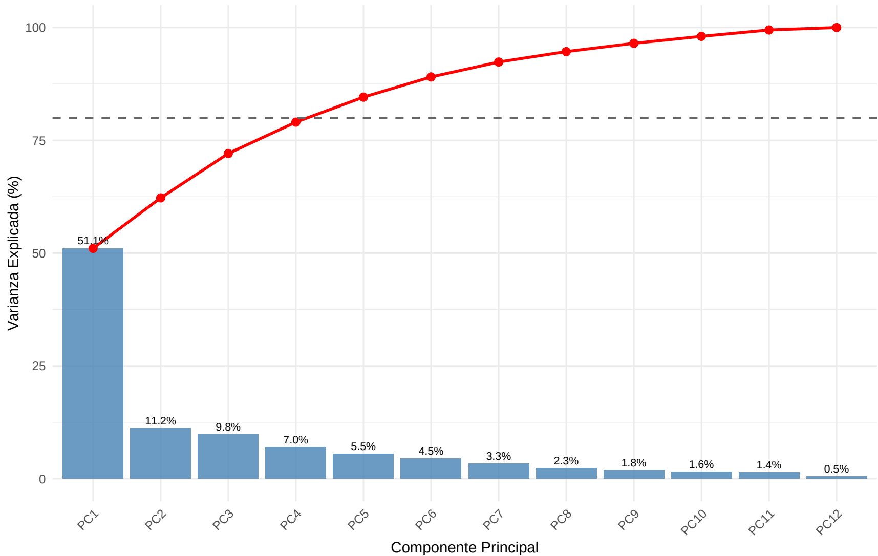
Scree Plot – Varianza Explicada por Componente Principal
