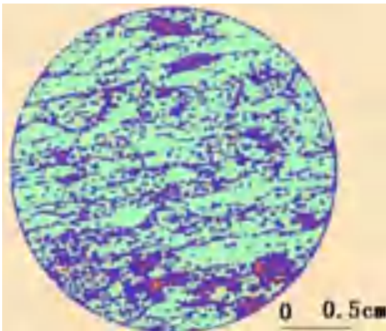
c) 片理
