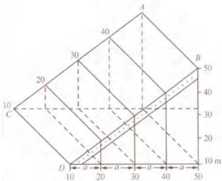
图 II-8 放线距
