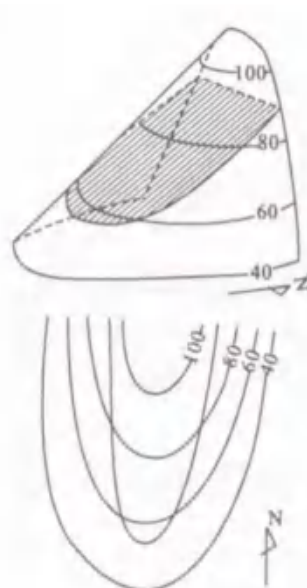
图 1-4 岩层倾向与地面坡向一致 岩层倾角小于地面坡角
