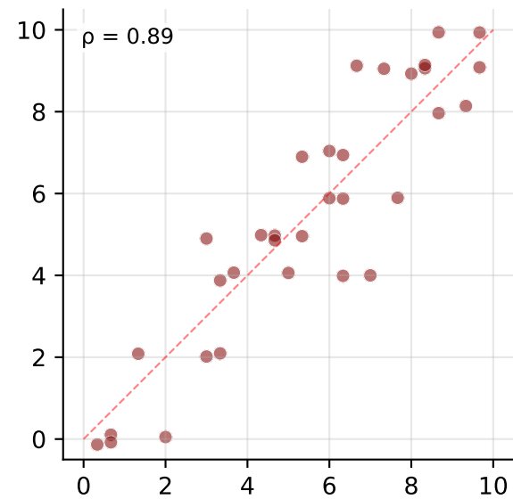
Coherence
