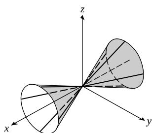
27. Circular cone
