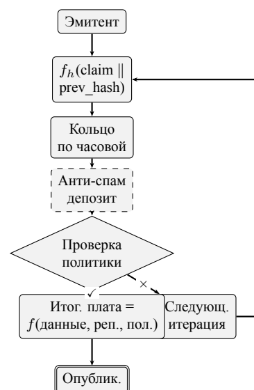
Figure 4: Протокол выбора верификатора. Анти-спам депозит опционален и может быть возвратным. Итоговая плата взимается только при принятии.
