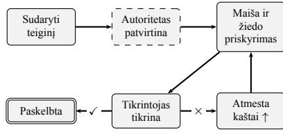
Figure 3: Teiginio gyvavimo ciklas su iteracijos kilpa.
