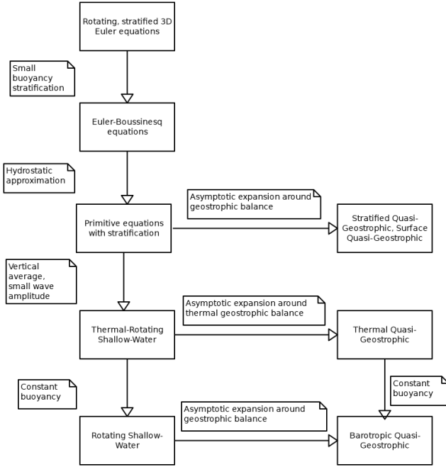
FIGURE 2 : Schéma de dérivation de quelques modèles GFD. Adapté de CRISAN et al., 2021 et Holmes
