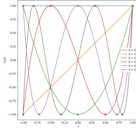
FIGURE 6 : Premiers polynomes de Chebyshev et points de Gauss-Lobatto
