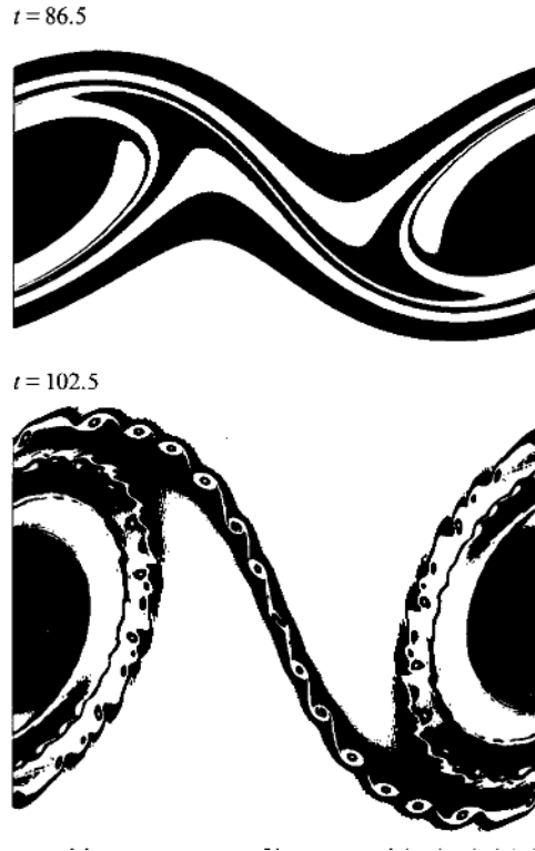
FIGURE 2 : Instabilité d'un filament de flottabilité. Tiré de HELD et al., 1995
