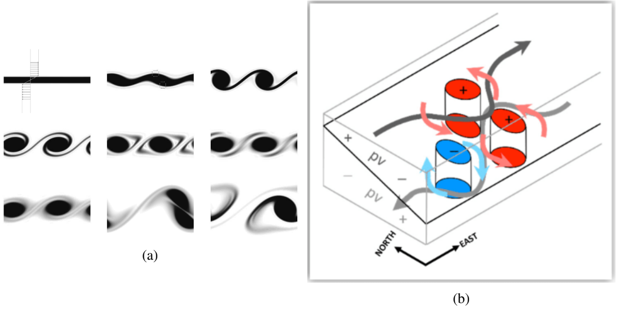
FIGURE 1 : 1a : instabilité barotrope (tiré de CUSHMAN-ROISIN et BECKERS, 2011); 1b : instabilité barocline (tiré de ILLIG et HALL, 2025)
