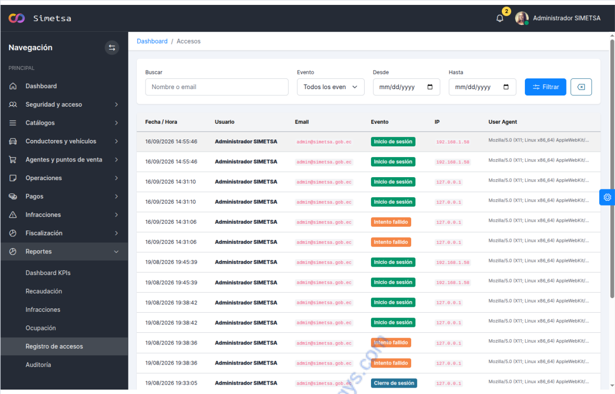
Figura 6. Registro de accesos al sistema.
