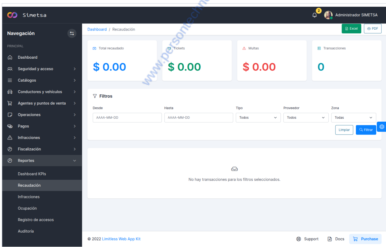
Figura 38. Reporte de recaudación con filtros y tabla paginada.
