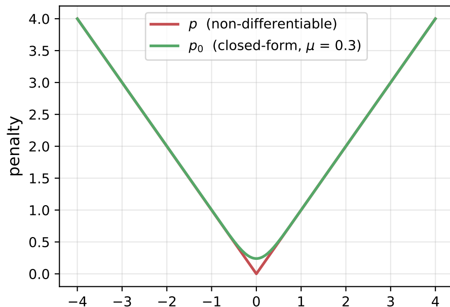
Lasso
