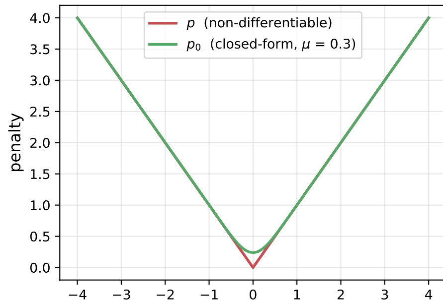
Lasso
