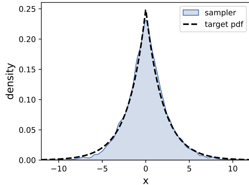
Subgradient LMC
