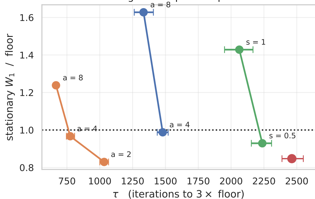
Target A: elliptical Laplace
