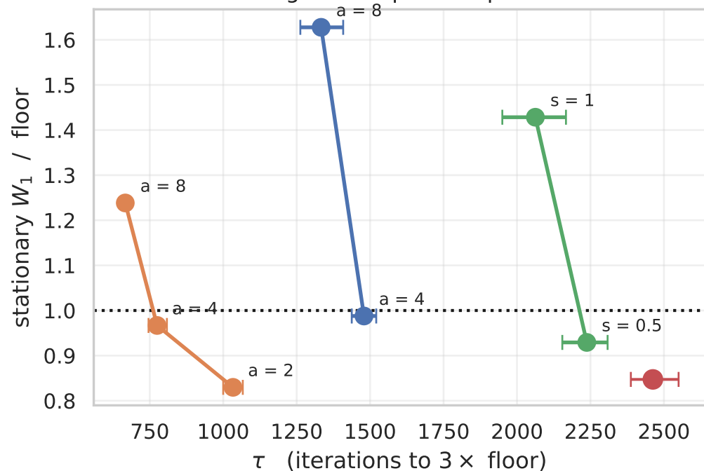
Target A: elliptical Laplace
