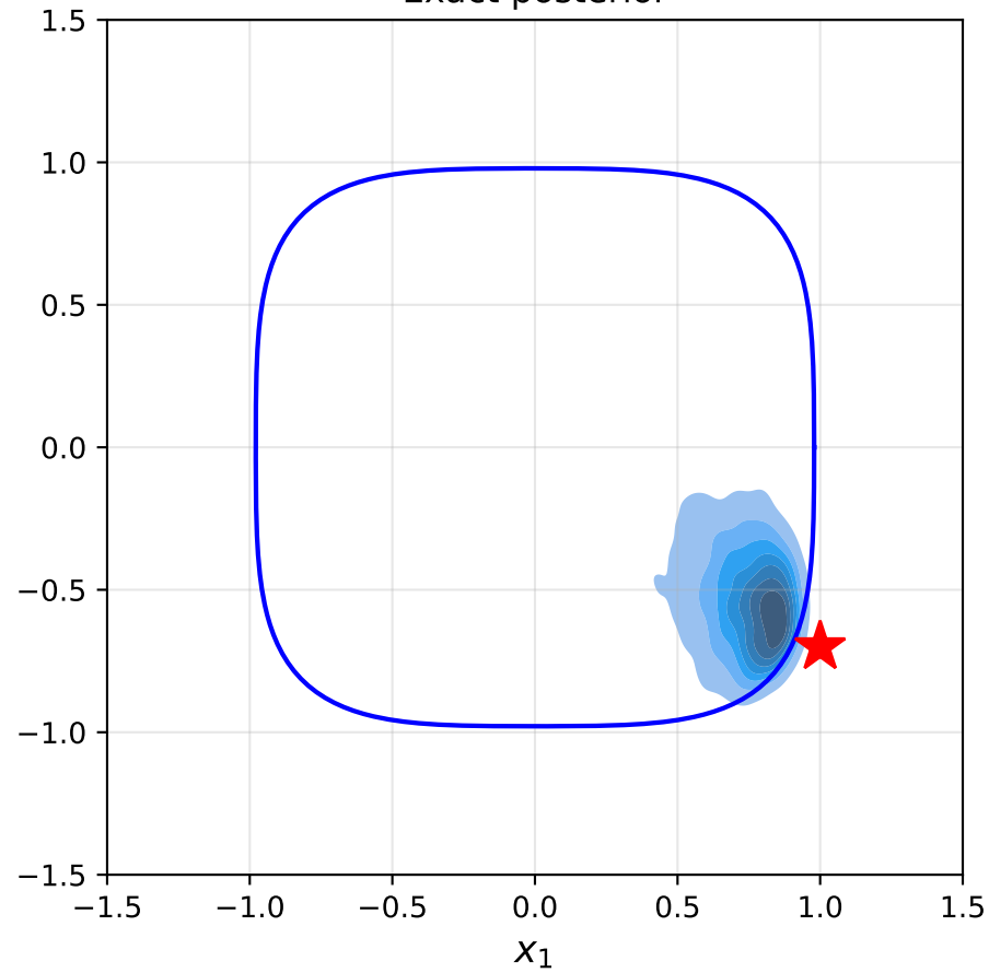
Exact posterior
