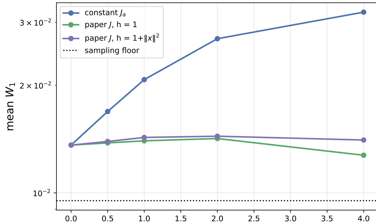
Ball \|x\|^2 \leq 1
