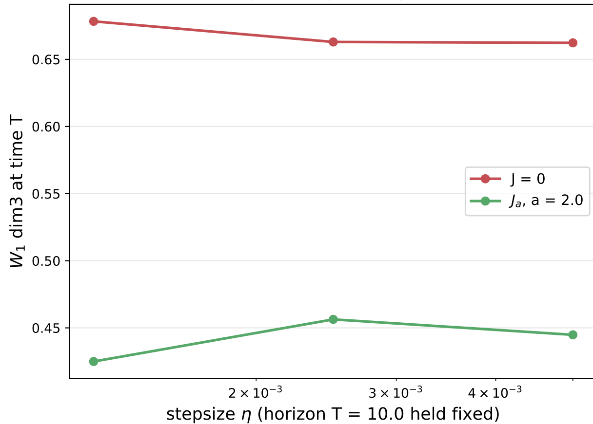
Target A: elliptical Laplace
