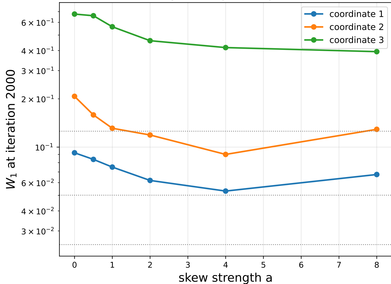
Target A: elliptical Laplace
